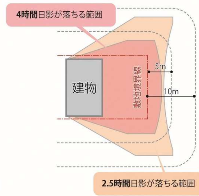
等時間日影のイメージ（平面図）
