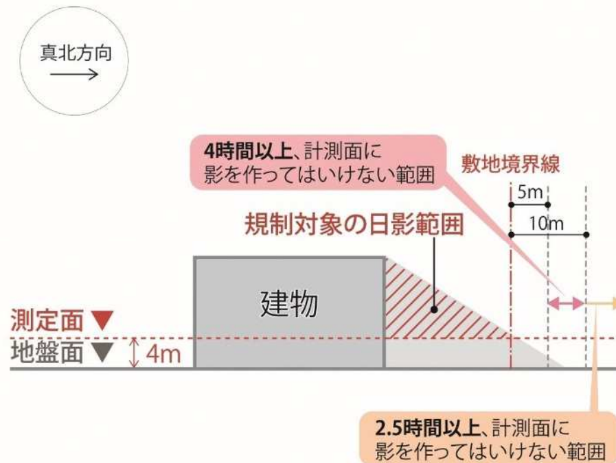
日影規制の考え方（立面図）
